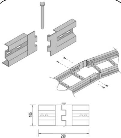
Horizontal Adjustable ปรับระดับแนวนอน
