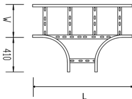
Horizontal Tee (HT)
