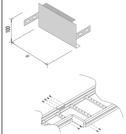
Reduce Connector ข้อลด
