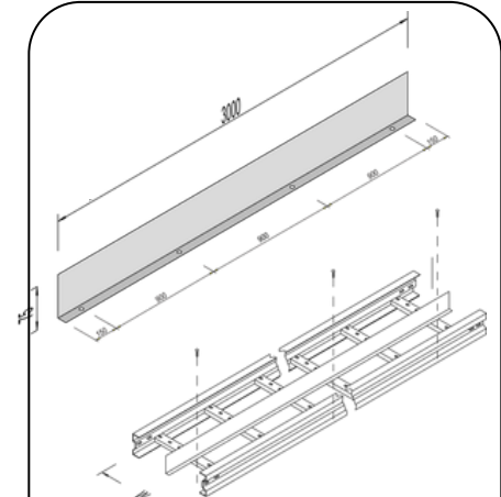
Separator แผ่นกั้นกลาง
