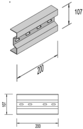
Splice Plate ข้อต่อตรง
