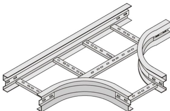
Horizontal Tee (HT)
