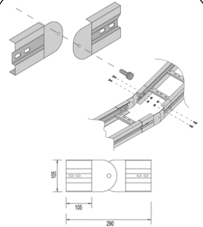
Vertical Adjustable ปรับระดับแนวตั้ง
