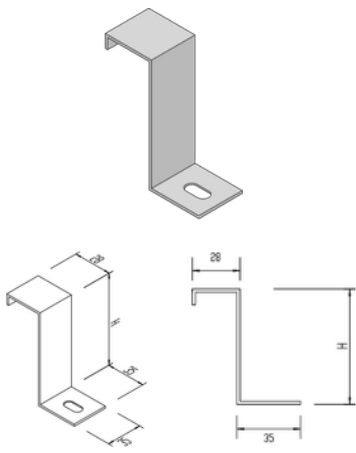
Hold-Down Clamp ข้อยึดราง
